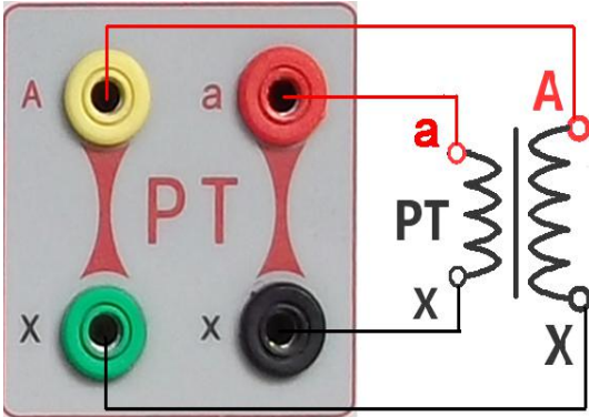
图 27，PT 变比极性（角差比差）接线图
