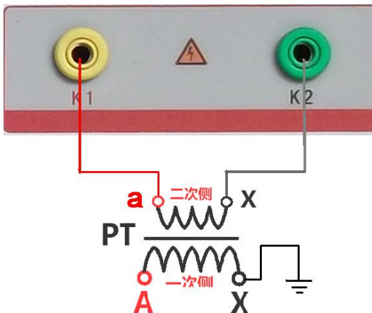
图 25，PT 励磁特性接线图
