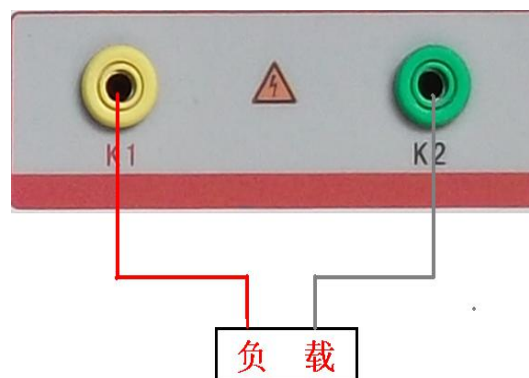
图 20, CT 二次负荷接线图
